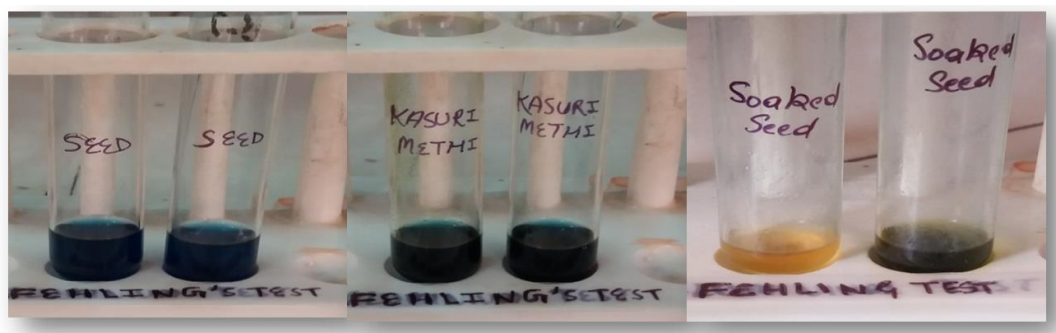
Figure 1: Fehling test
