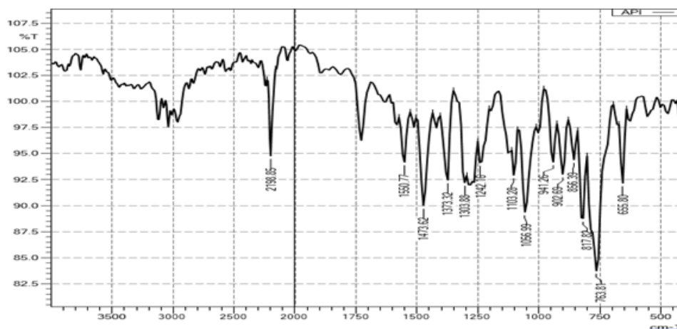
Fig.no.4. IR spectra of Luliconazole (API)
