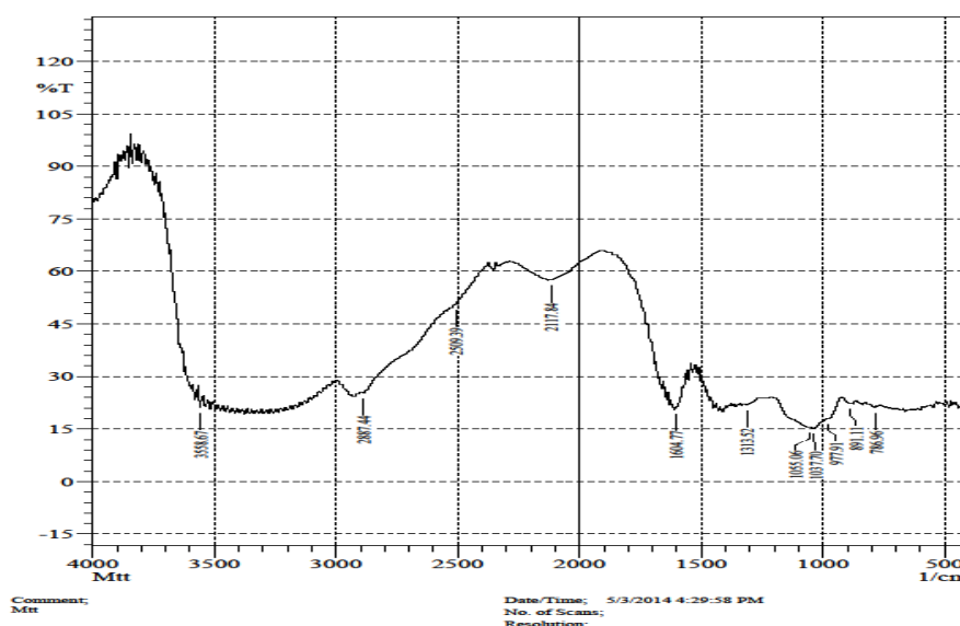
Fig1. IR spectra of Mardi ( terminaliatomentosa) gum
