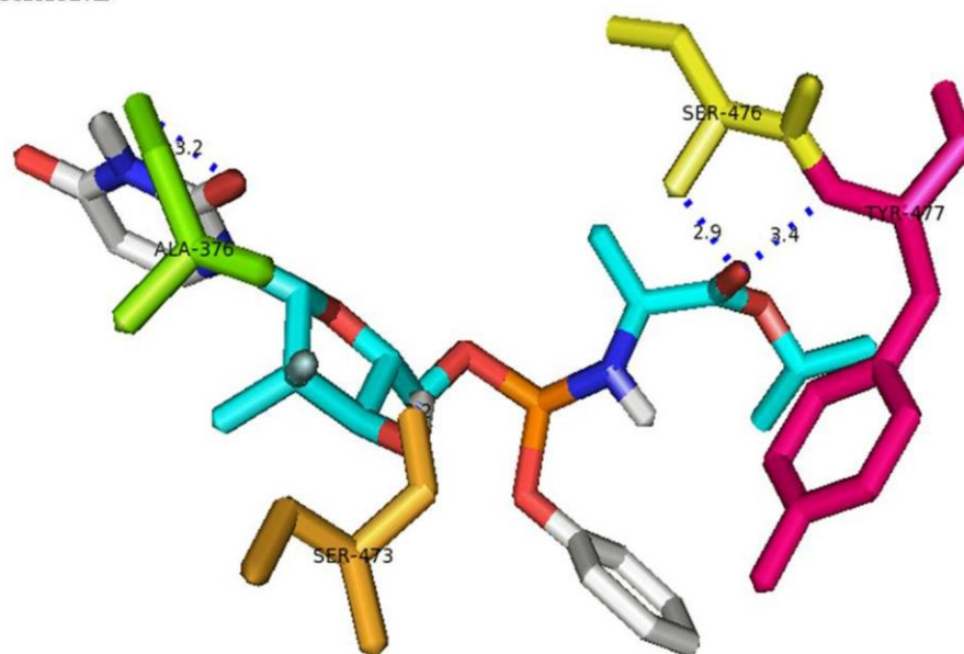
Sofosbuvir
